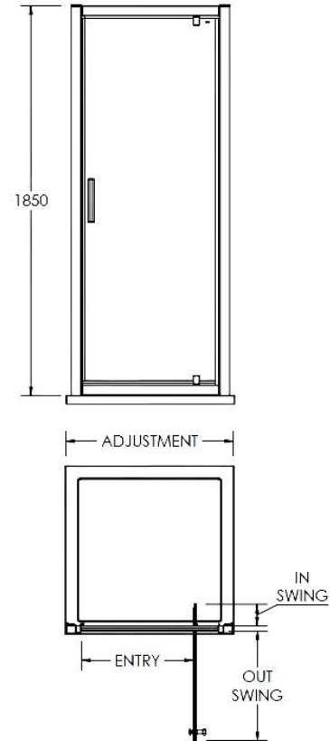
Pacific Pivot Door Enclosure
